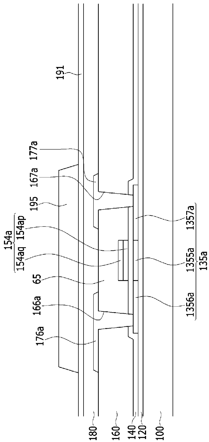
FIG. 28
